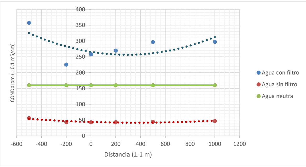
Gráfico 3.2: Comparación de la conductividad de las muestras con y sin biofiltro de conchas de abanico.
