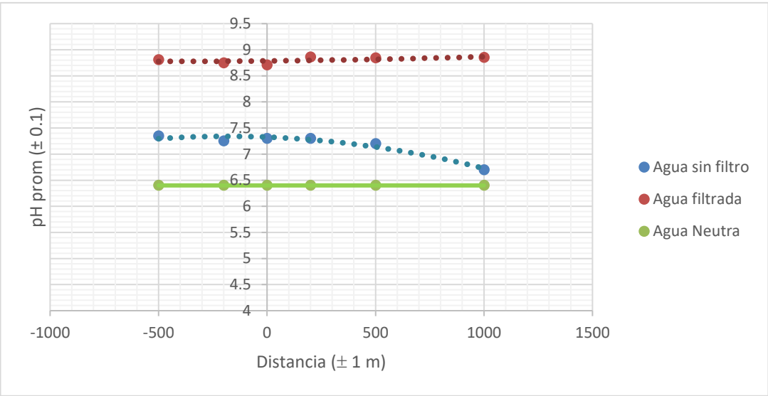
Gráfico 3.1: Comparación del pH de las muestras con y sin biofiltro de conchas de abanico.
