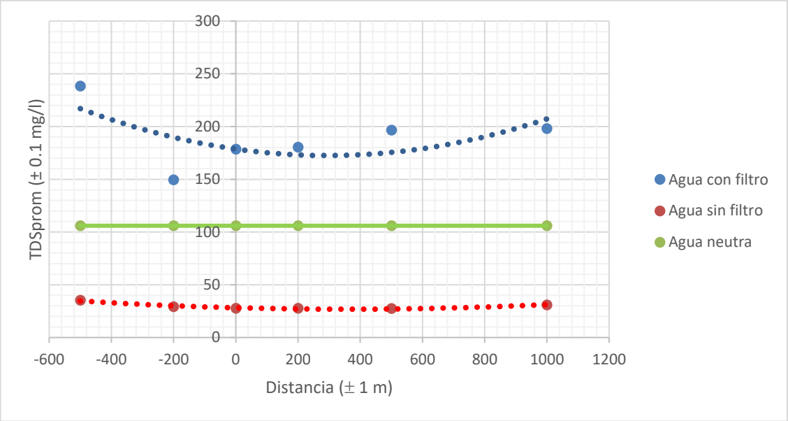
Gráfico 3.3: Comparación del TDS de las muestras con y sin biofiltro de conchas de abanico.
